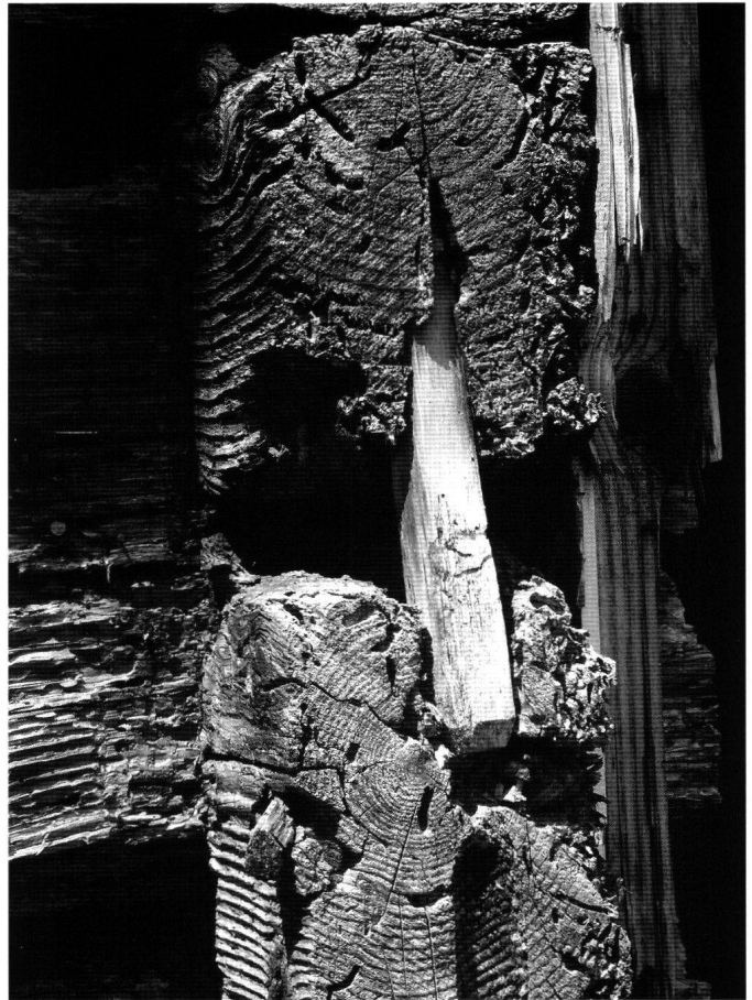
Abb. 9: Südfassade, sekundär abgesägte Vorstösse mit eckigem Holzdübel.
