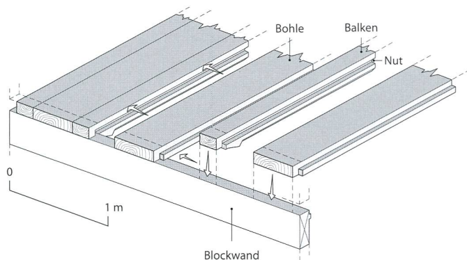
Abb. 6 Bohlen-Balken-Decke.
